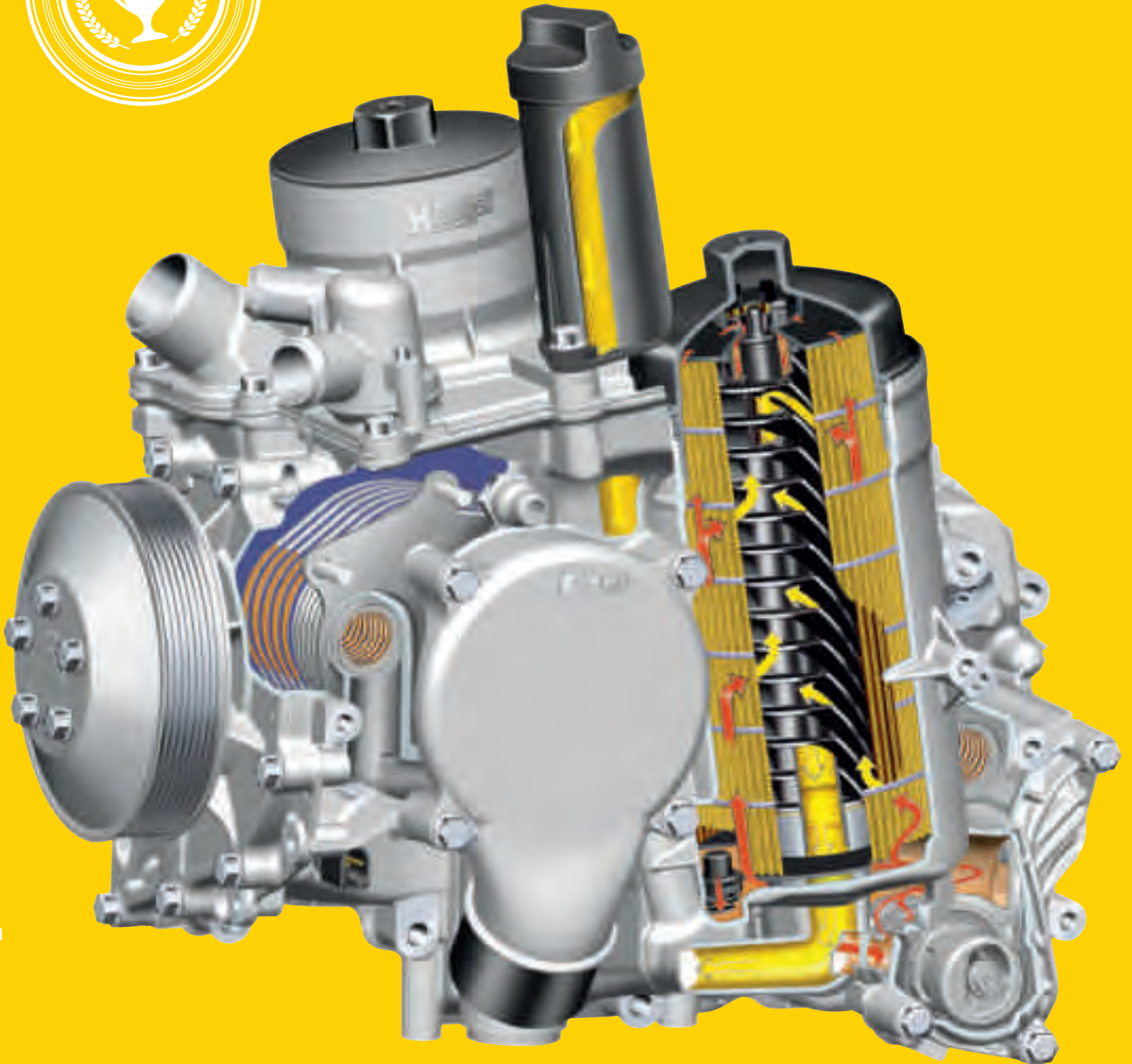
— Módulo de administración de fluidos para camiones de Daimler Truck Group
